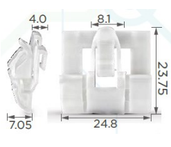
Honda Door Window
